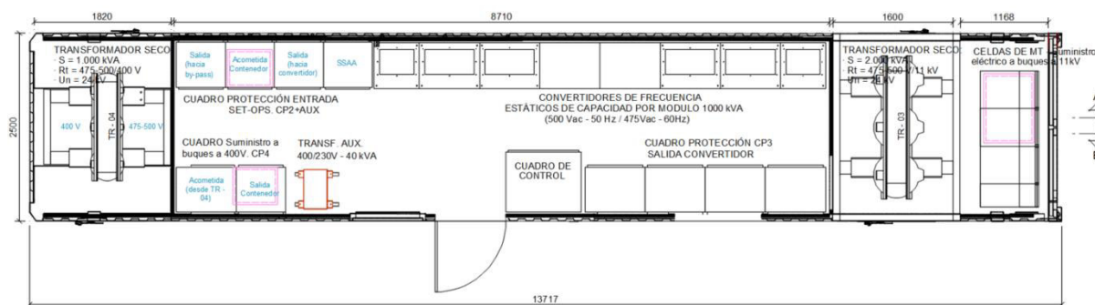
Figura 21. Planta orientativa de la Subestación Transformadora SET-OPS
