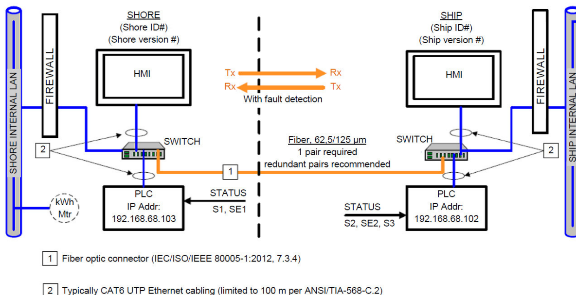
Figura 24. Esquema general de Comunicación de datos
