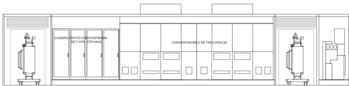
Figura 22. Sección orientativa de la Subestación Transformadora SET-OPS
