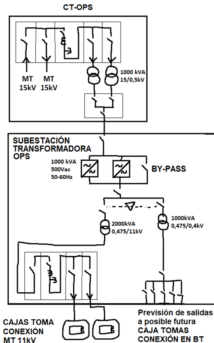
Figura 10. Esquema conceptual de la Solución Adoptada para la electrificación de los Muelles de Poniente
