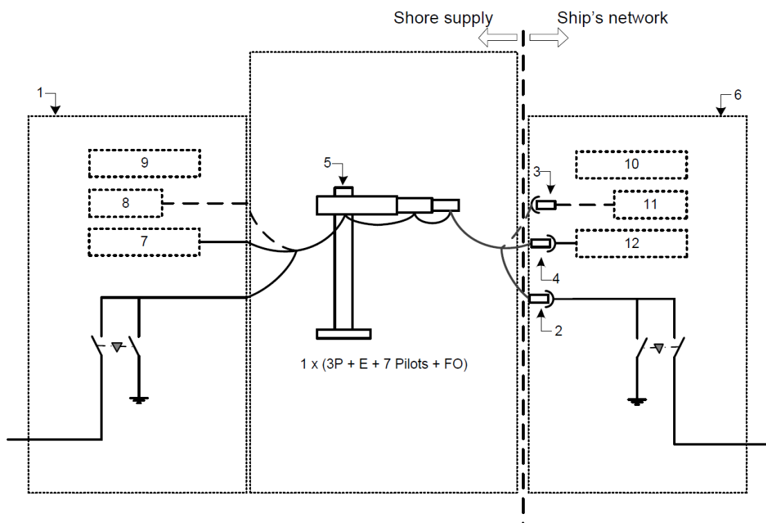
Figura 8. Esquema general de la distribución a buques en MT
