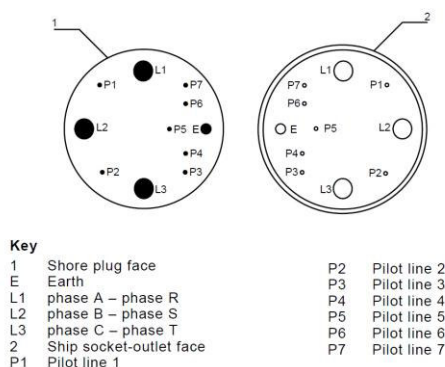
Figura 11. Conector Trifásico para red MT según la IEC/ISO/IEEE 80005-1 "(Figure B.3 – Three-phase plug and socket-outlet contact assignment)"
