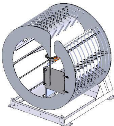
Figura 35. Carrete de almacenamiento
