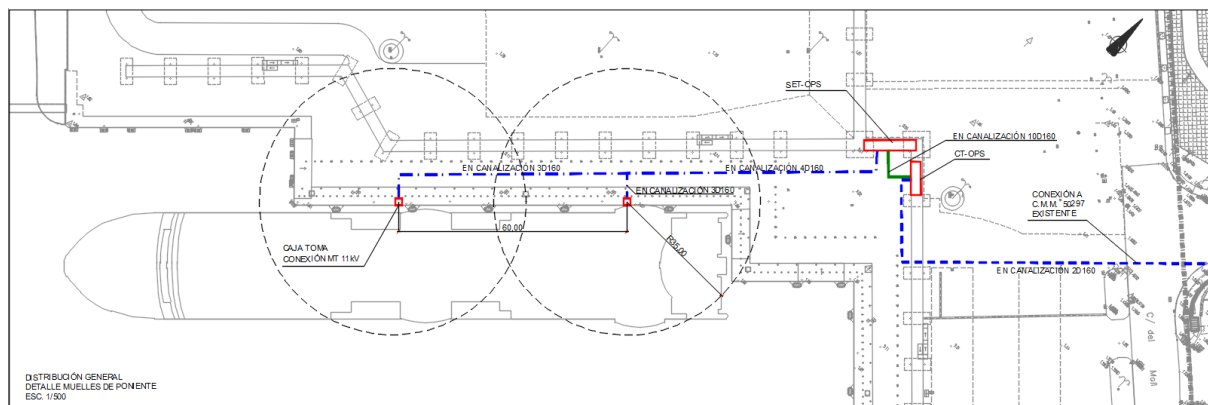
Figura 4. Distribución eléctrica a cajas de tomas situadas a borde de muelle
