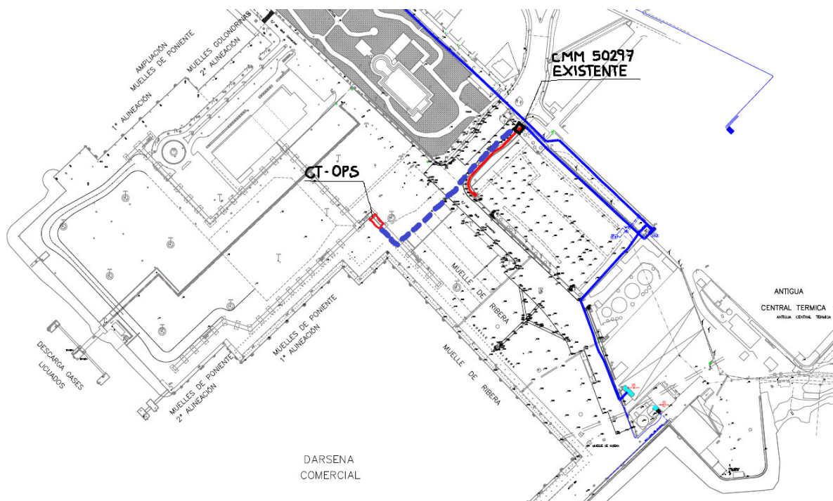
Figura 7. Propuesta acometida en MT 15kV a Centro de Transformación OPS
