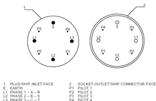
Figura 12. Conector Trifásico para red BT según la IEC/ISO/IEEE 80005-3 (Figure C.2 - Power plug and socket-outlet contact assignment)
