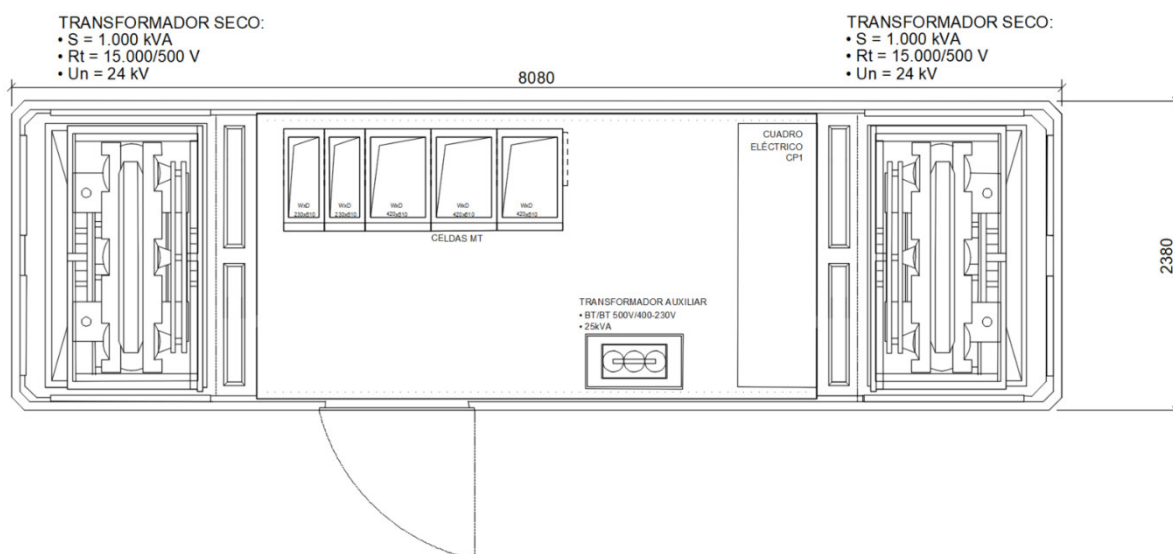
Figura 15. Planta orientativa Centro de Transformación CT-OPS
