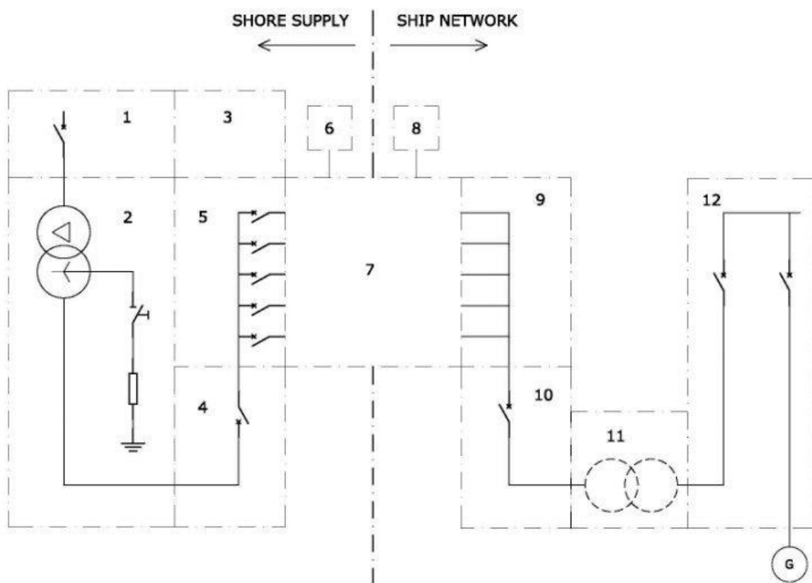
Figura 9. Esquema general de la distribución a buques en BT
