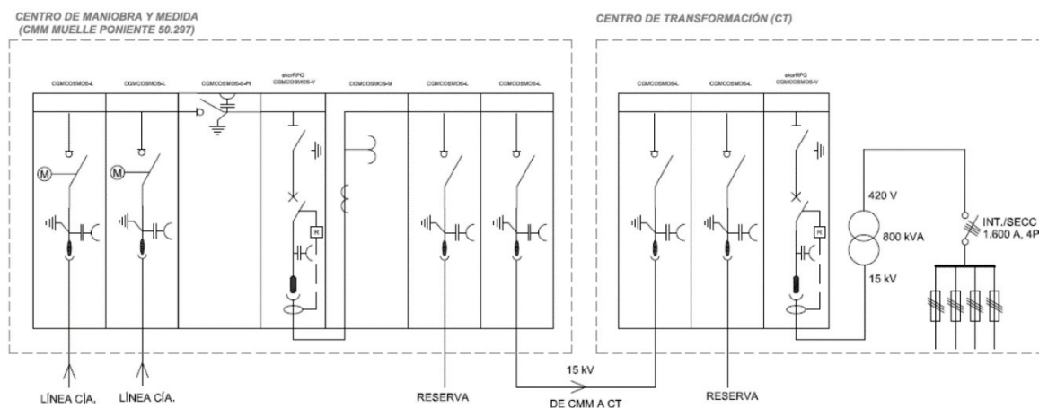
Figura 6. Esquema eléctrico CMM Muelle de Poniente 50297 y CT
