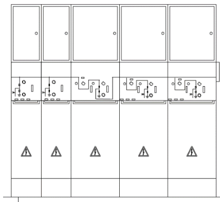
Figura 19. Alzado orientativo apartamento de MT del Centro de Transformación CT-OPS
