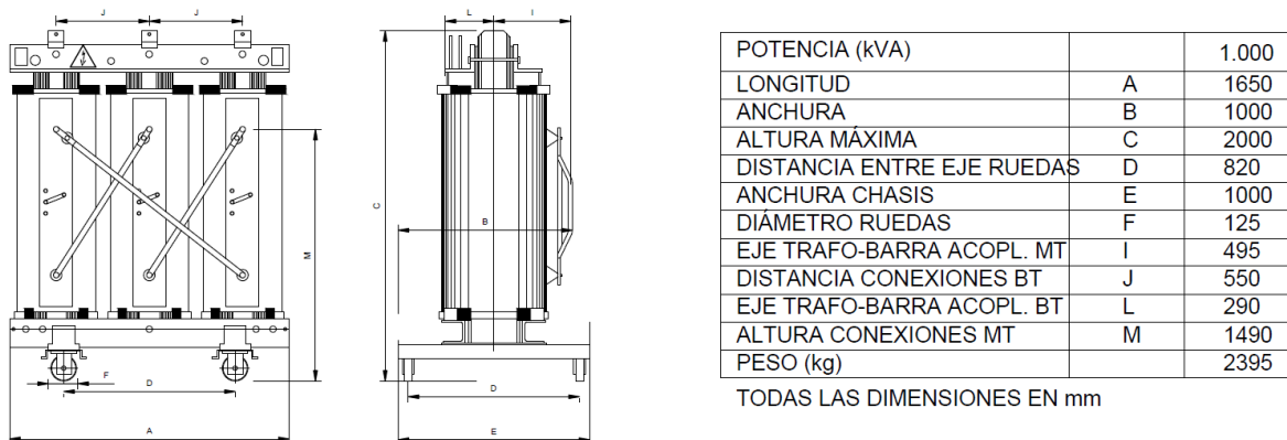
Figura 20. Dimensiones orientativas transformador del Centro de Transformación CT-OPS
