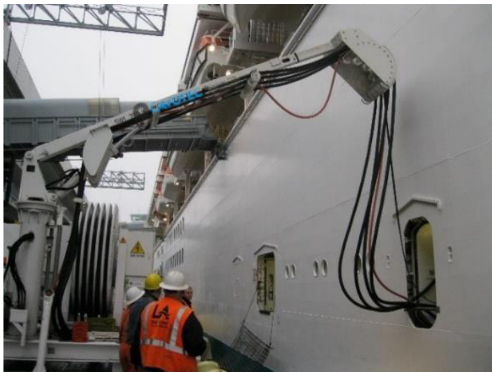
Figura 30. Reposicionar la grúa para dejar holgura en los cables de conexión
