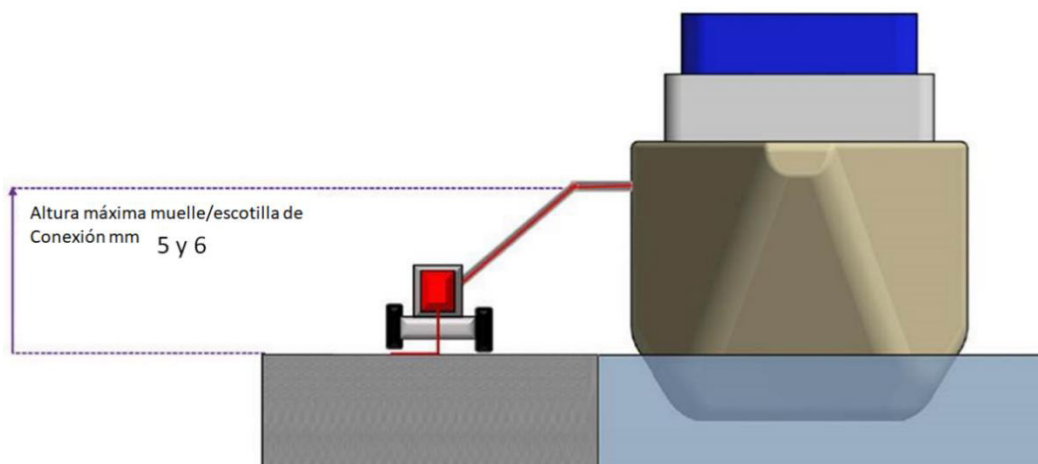
Figura 14. Distancias entre Sistema de suministro eléctrico y barco (Vista lateral)
