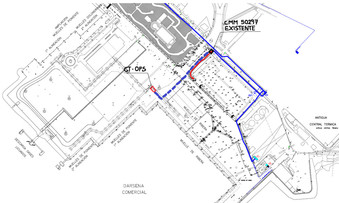
Figura 3. Propuesta acometida en MT 15kV a Centro de Transformación OPS
