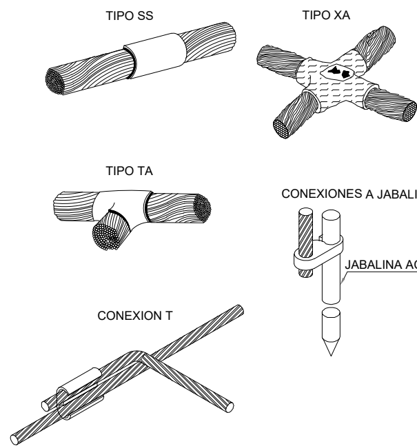
DETALLES TIPO SOLDADURA. SIN ESCALA
