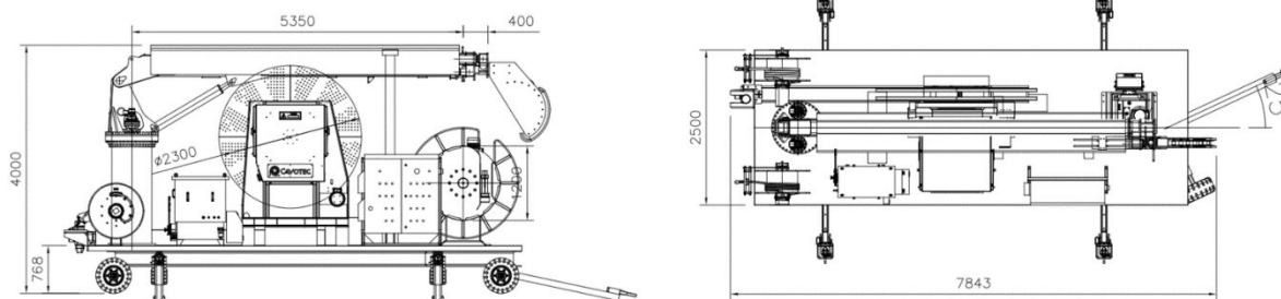
Figura 25. Alzado y Planta de la Unidad de Gestión de Cable
