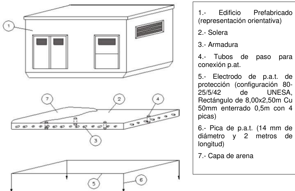
Figura 17. Detalle constructivo solera hormigón armado CT
