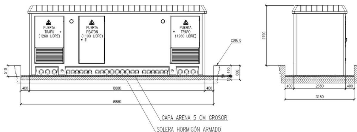
Figura 17. Detalle constructivo solera hormigón armado CT
