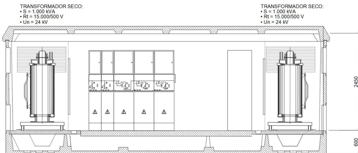
Figura 16. Sección orientativa Centro de Transformación CT-OPS
