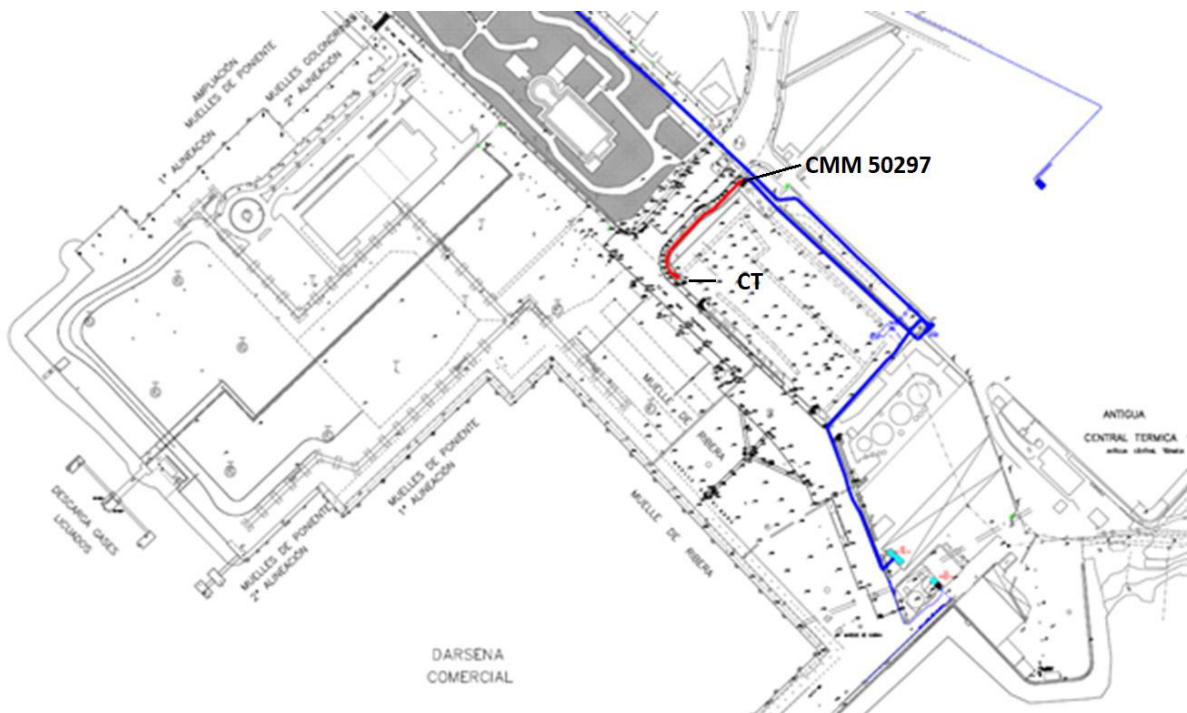
Figura 5. Plano Servicios Existentes Media Tensión
