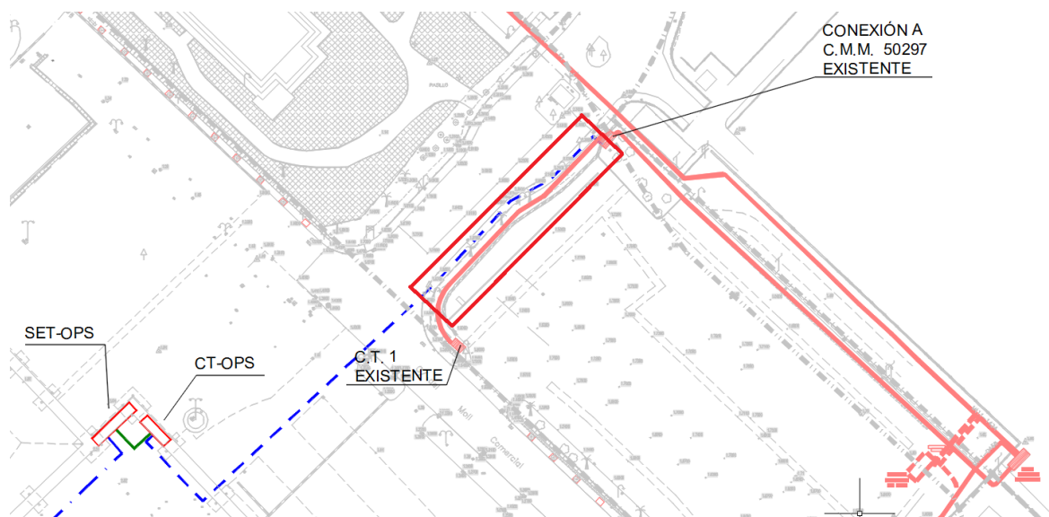
Figura 41. Servicios afectados. Paralelismo entre canalizaciones de MT
