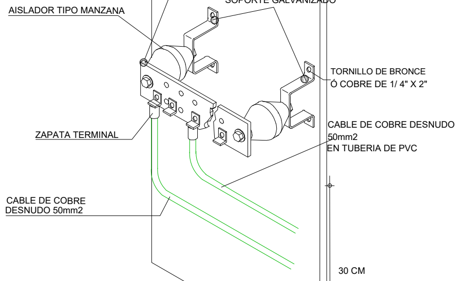
DETALLE EMBARRADO TIERRAS PERSPECTIVA. SIN ESCALA
