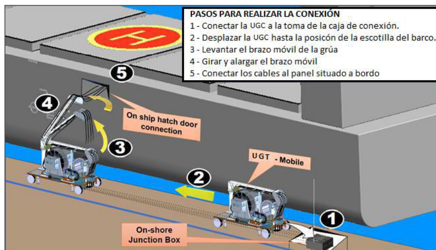
Figura 27. Procedimiento de conexión de la UGC
