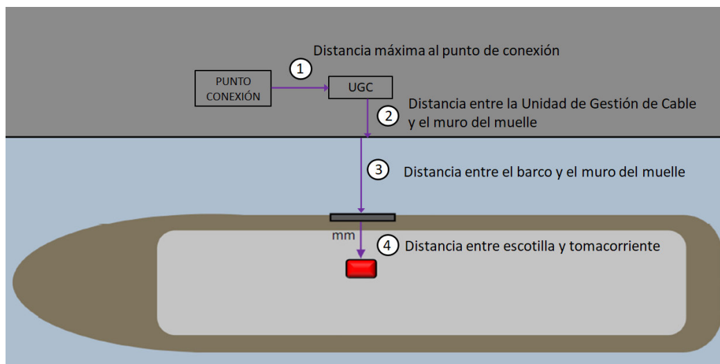
Figura 13. Distancias entre Sistema de suministro eléctrico y barco (Planta)
