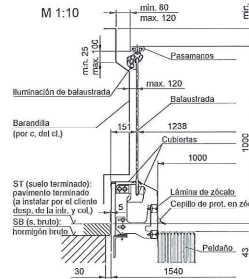
Corte A-A
