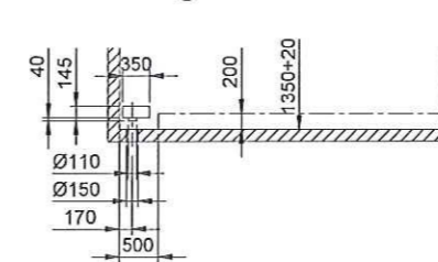
Separador de aceite con desagüe
