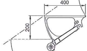
Detalle peldaño M 1:10
