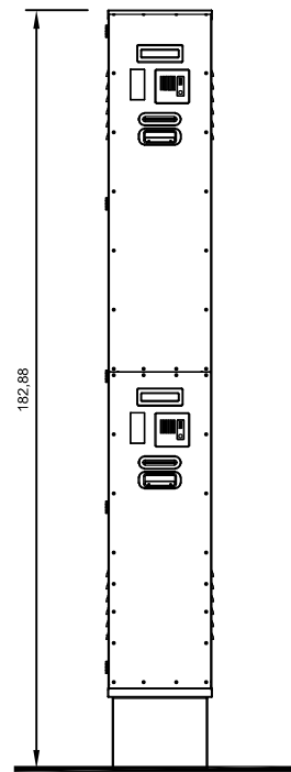
Poste peana vial de entrada
