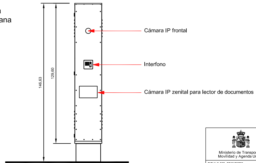
Poste peana Control remoto puerta corredera entrada y salida
