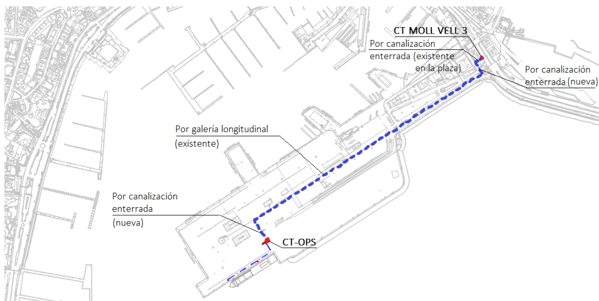
Figura 14. Propuesta acometida en MT 15kV de CT MOLL VELL 3 a Centro de Transformación OPS
