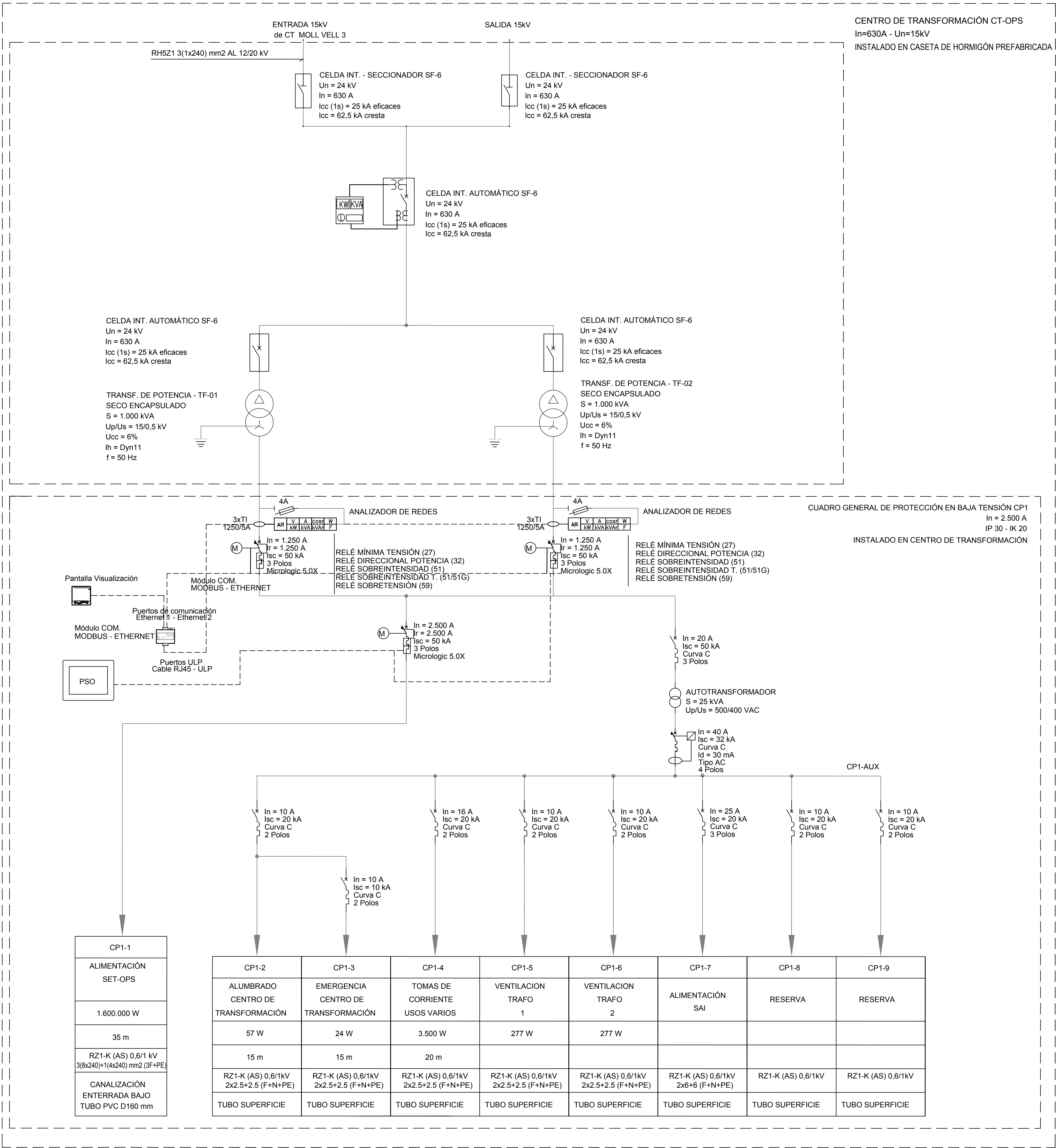
DETALLE 1. CUADRO GENERAL DE PROTECCIÓN EN BAJA TENSION DE SALIDA CP1 ESCALA 1:20
