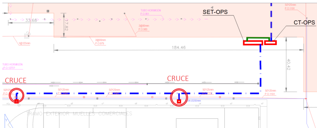
Figura 48. Servicios afectados. Cruce con instalaciones de Agua Potable y Canalizaciones de Servicios
