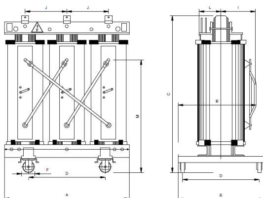
Figura 27. Dimensiones orientativas transformador del Centro de Transformación CT-OPS
