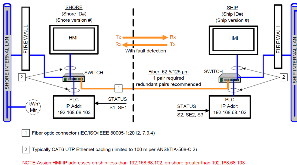
Figura 31. Esquema general de Comunicación de datos
