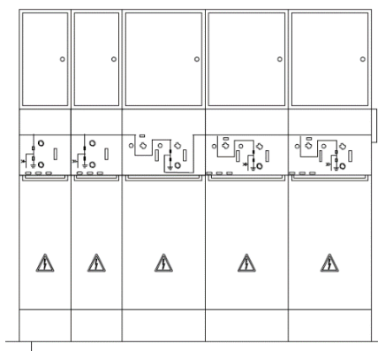
Figura 26. Alzado orientativo apartamento de MT del Centro de Transformación CT-OPS
