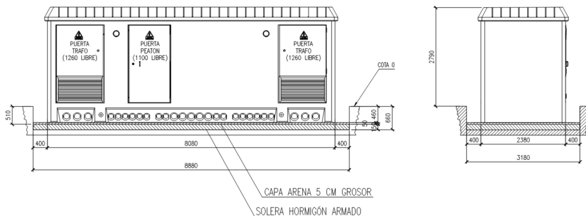
Figura 25. Vistas laterales detalle cimentación CT
