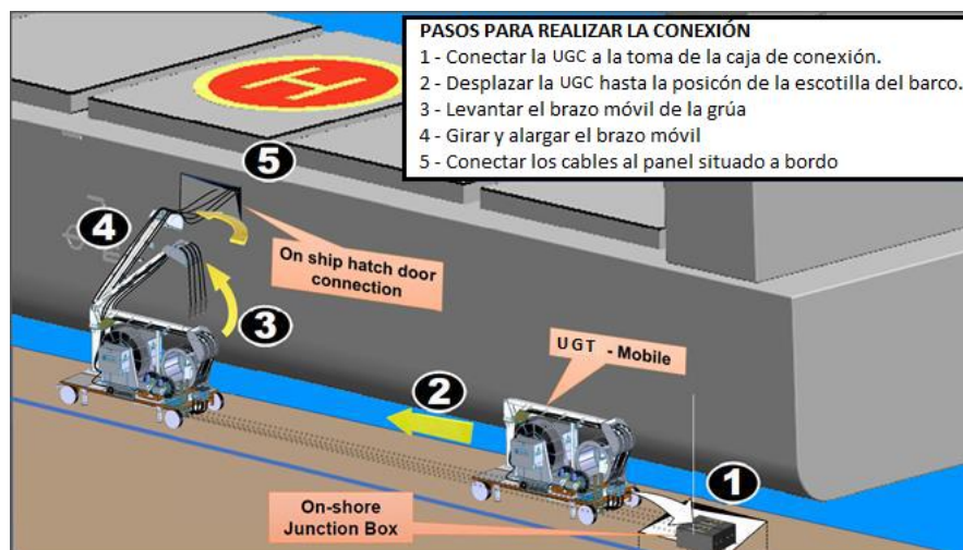
Figura 34. Procedimiento de conexión de la UGC
