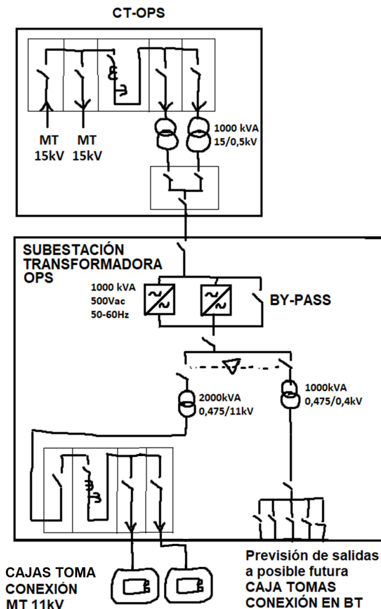
Figura 17. Esquema conceptual de la Solución Adoptada para la electrificación de los Muelles Comerciales
