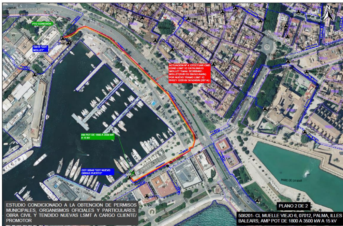
Figura 8. Actuaciones propuestas por la compañía (2 de 2) En rojo conductor existente a sustituir. En naranja nuevo conductor RH5Z1 12/20 kV 3x1x240/AI
