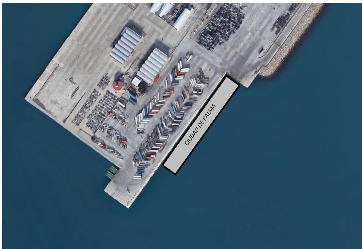
Figura 4. Posición de atraque del Ferry 'Ciudad de Palma' en los Muelles Comerciales del Puerto de Palma
