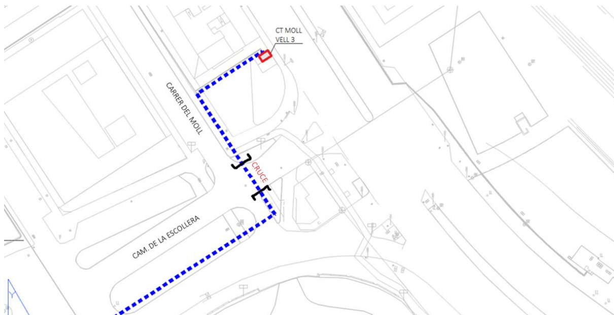
Figura 46. Cruce del Camino de la Escollera
