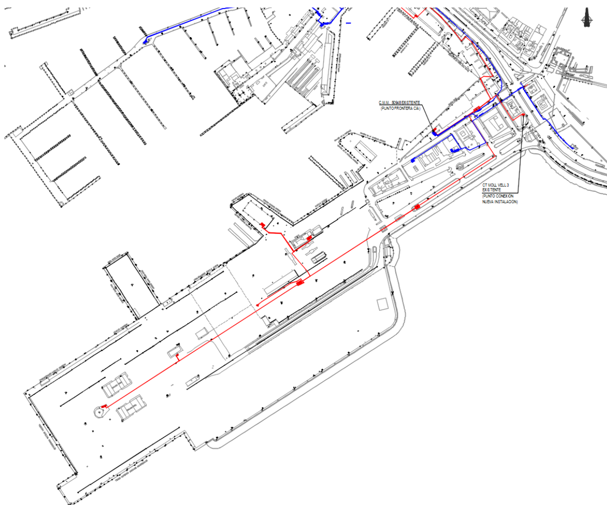
Figura 5. Plano Servicios Existentes Media Tensión
