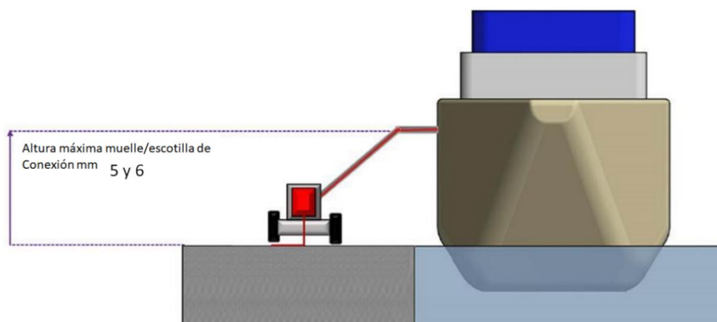
Figura 21. Distancias entre Sistema de suministro eléctrico y barco (Vista lateral)
