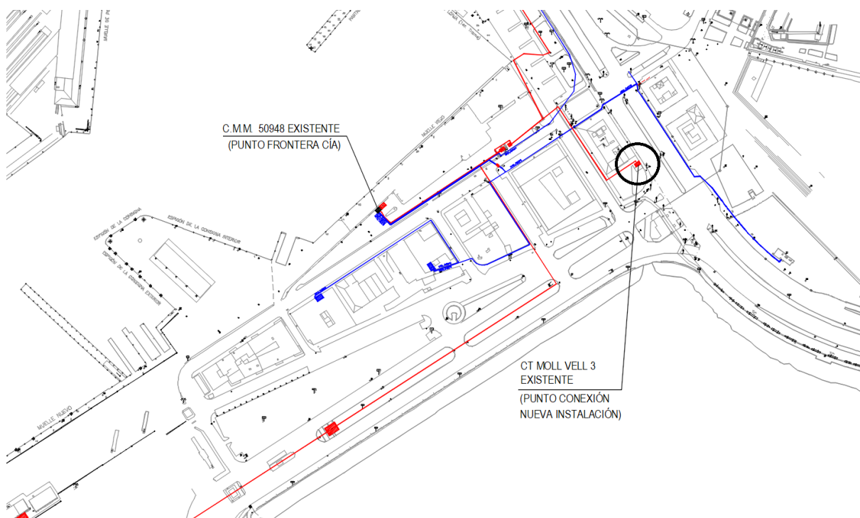
Figura 12. Redes de MT existentes en la zona. Endesa (en azul) y APB (en rojo)
