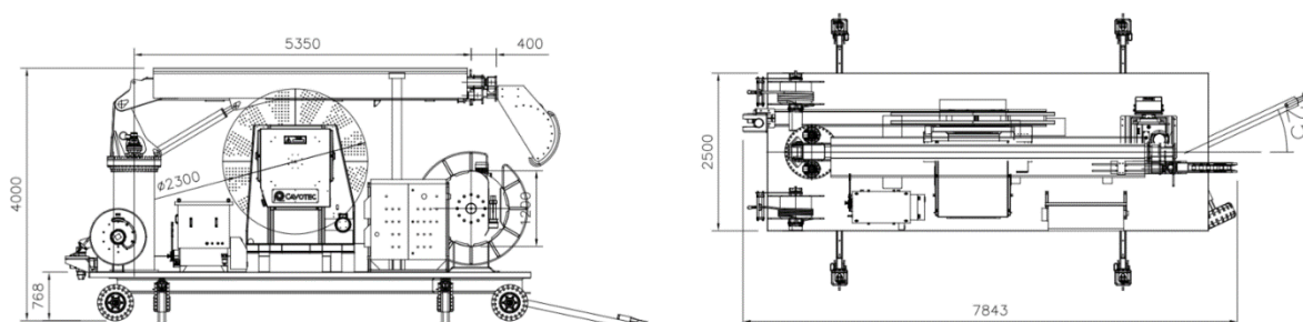
Figura 32. Alzado y Planta de la Unidad de Gestión de Cable
