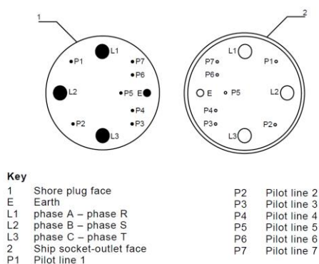
Figura 18. Conector Trifásico para red MT según la IEC/ISO/IEEE 80005-1 "(Figure B.3 – Three-phase plug and socket-outlet contact assignment)"
