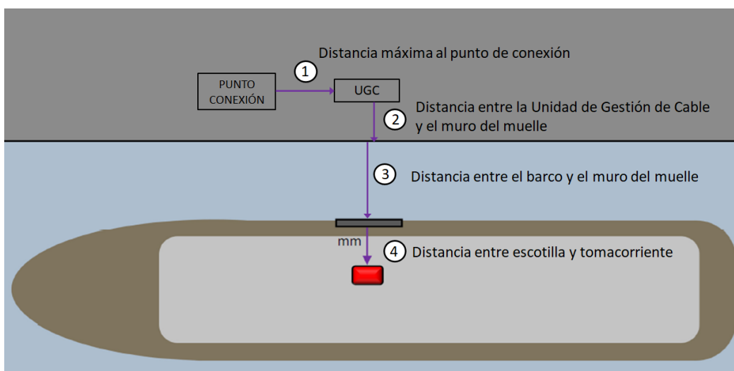
Figura 20. Distancias entre Sistema de suministro eléctrico y barco (Planta)
