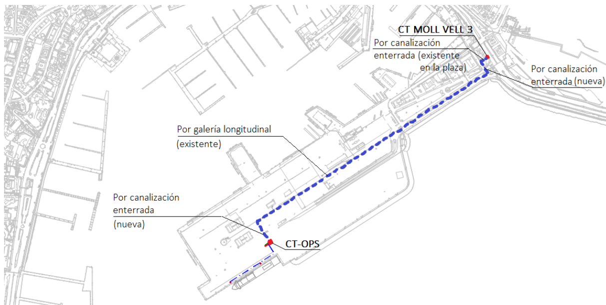
Figura 3. Propuesta acometida en MT 15kV a Centro de Transformación OPS
