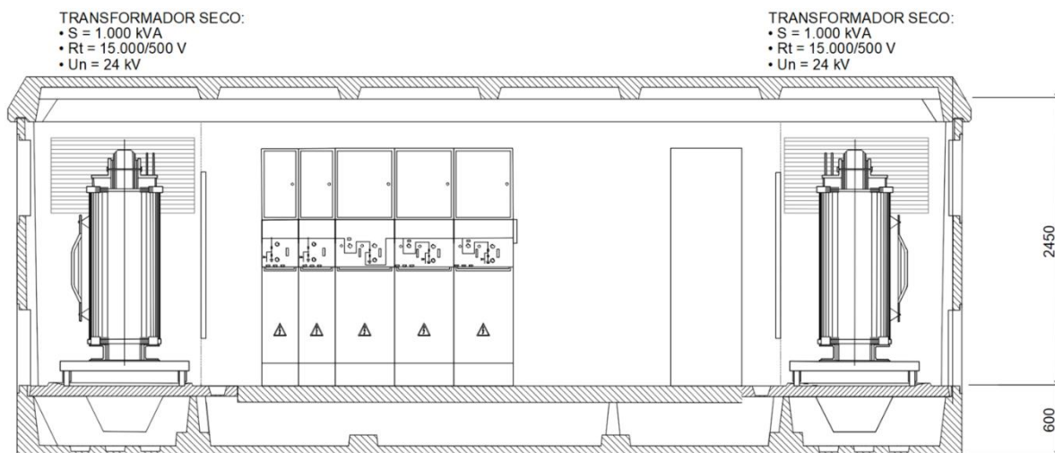
Figura 23. Sección orientativa Centro de Transformación CT-OPS
