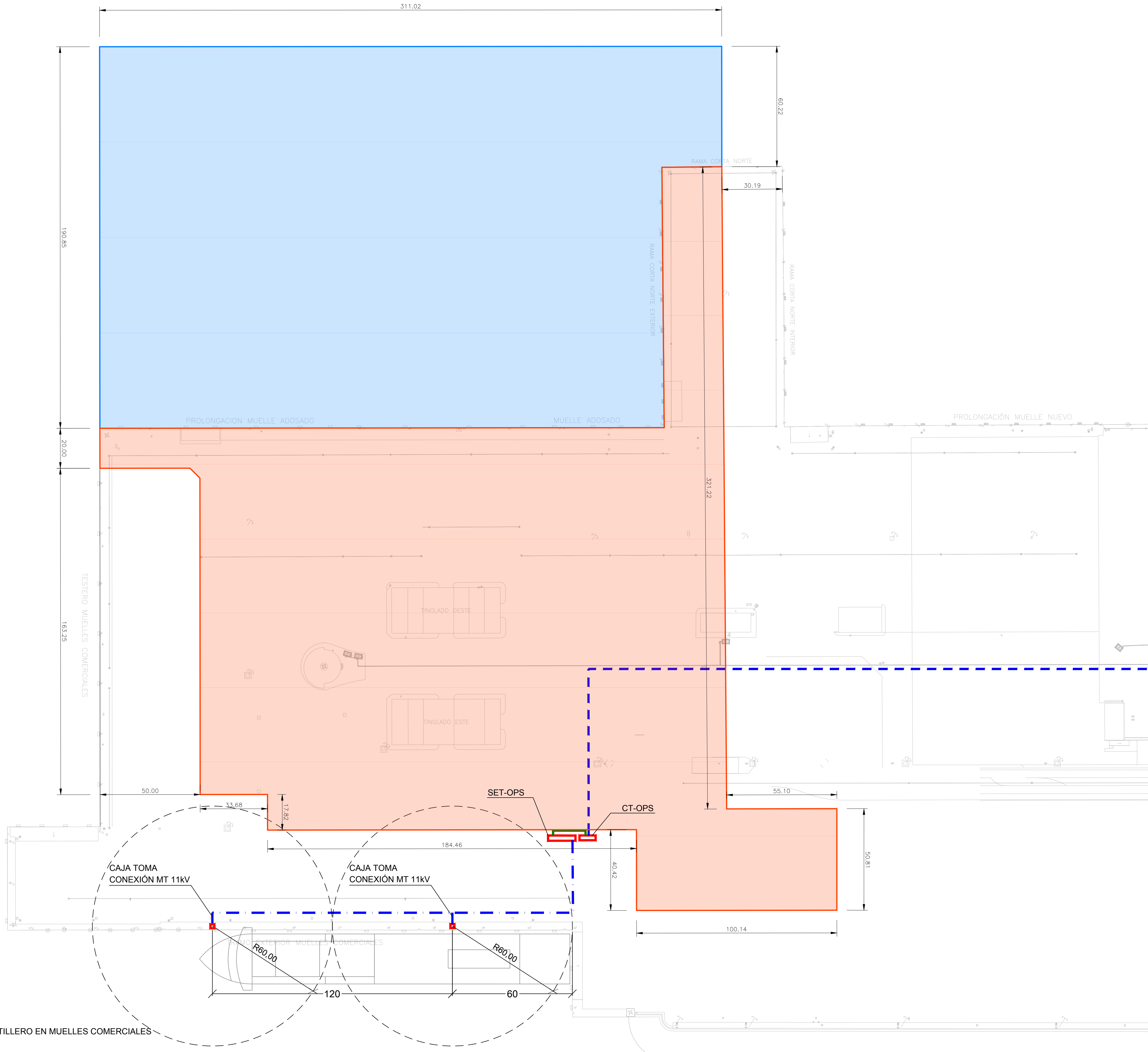
LOCALIZACIÓN GENERAL DETALLE PLANTA S/E
