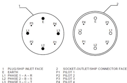
Figura 19. Conector Trifásico para red BT según la IEC/ISO/IEEE 80005-3 (Figure C.2 - Power plug and socket-outlet contact assignment)
