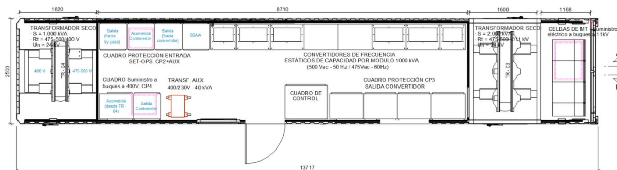
Figura 28. Planta orientativa de la Subestación Transformadora SET-OPS
