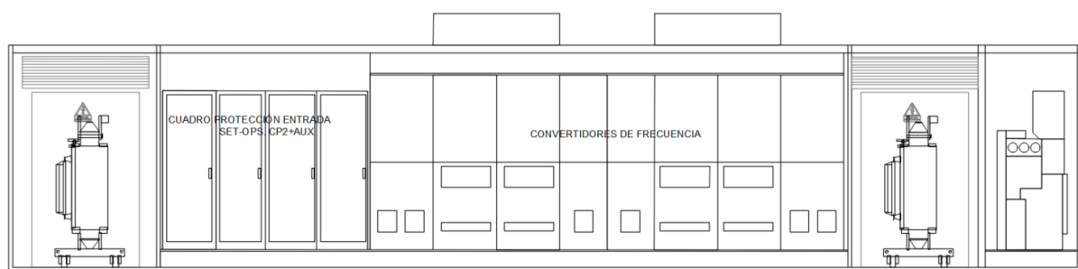
Figura 29. Sección orientativa de la Subestación Transformadora SET-OPS
