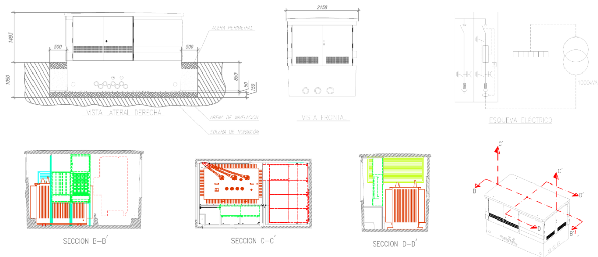
Figura 13. CT MOLL VELL 3
