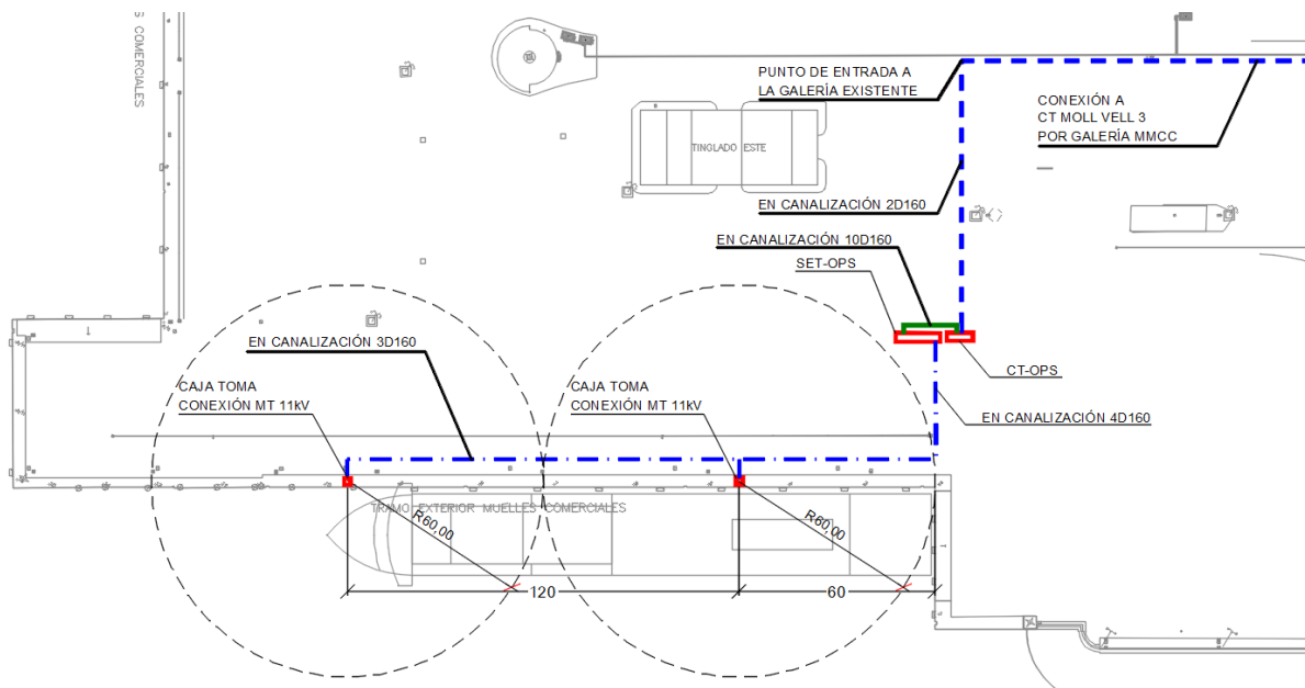
Figura 4. Distribución eléctrica a cajas de toma de MT situadas a borde de muelle
