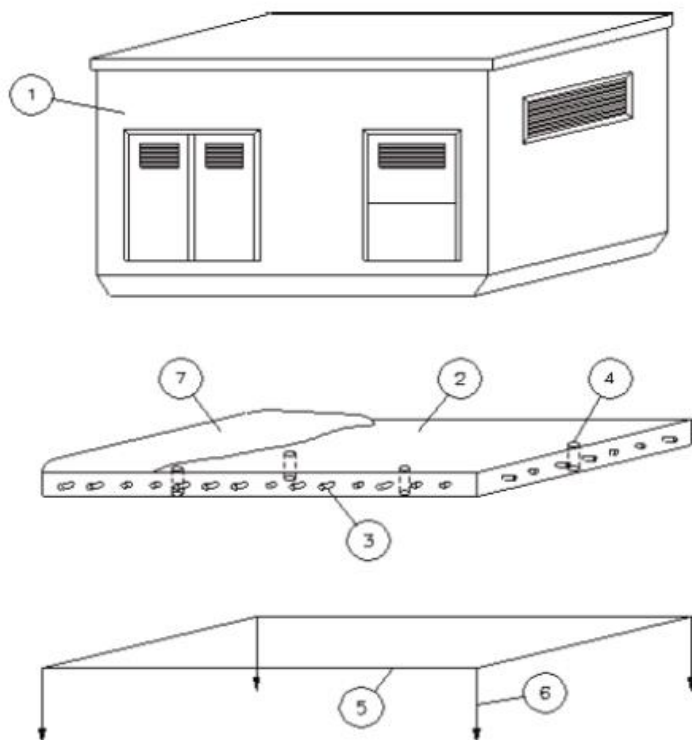
Figura 24. Detalle constructivo solera hormigón armado CT
