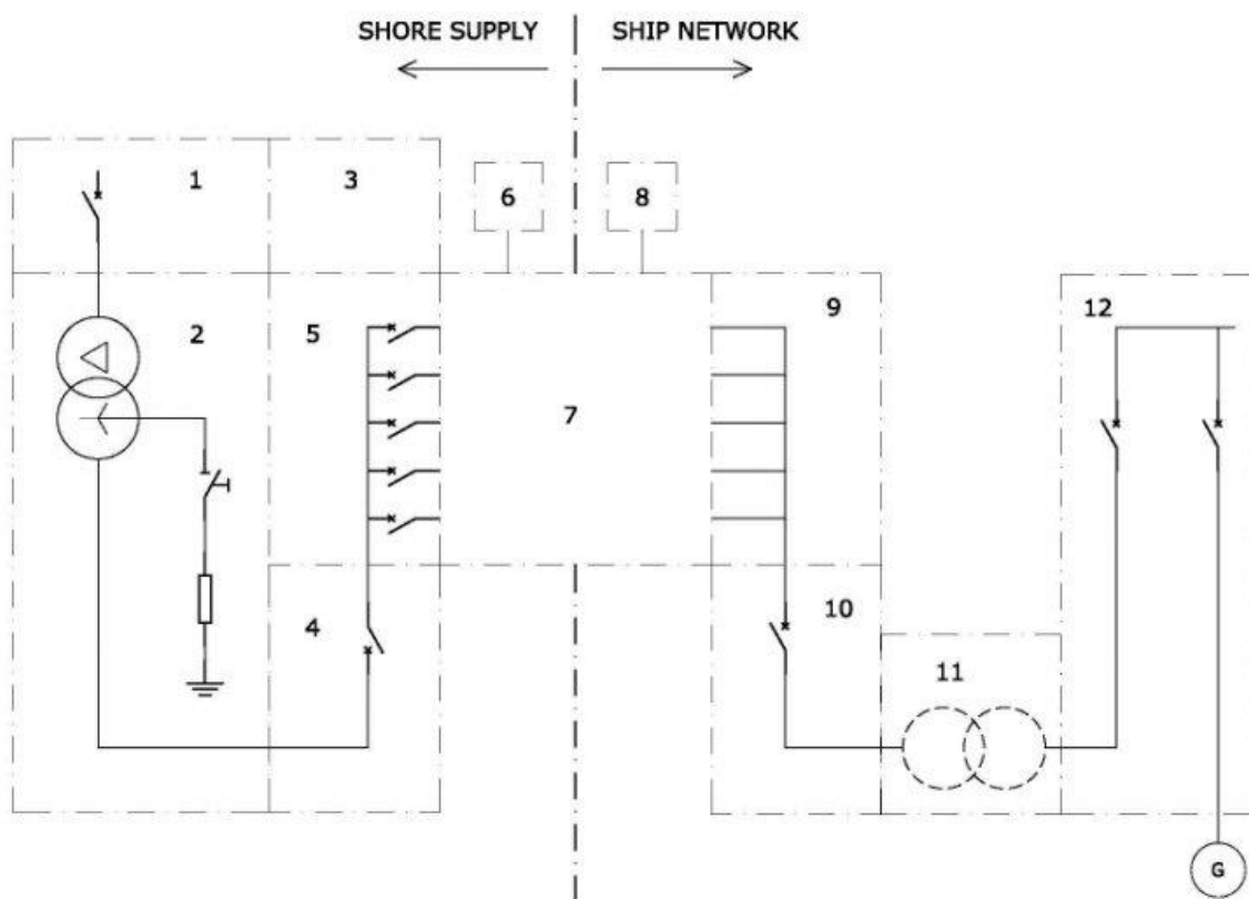
Figura 16. Esquema general de la distribución a buques en BT
