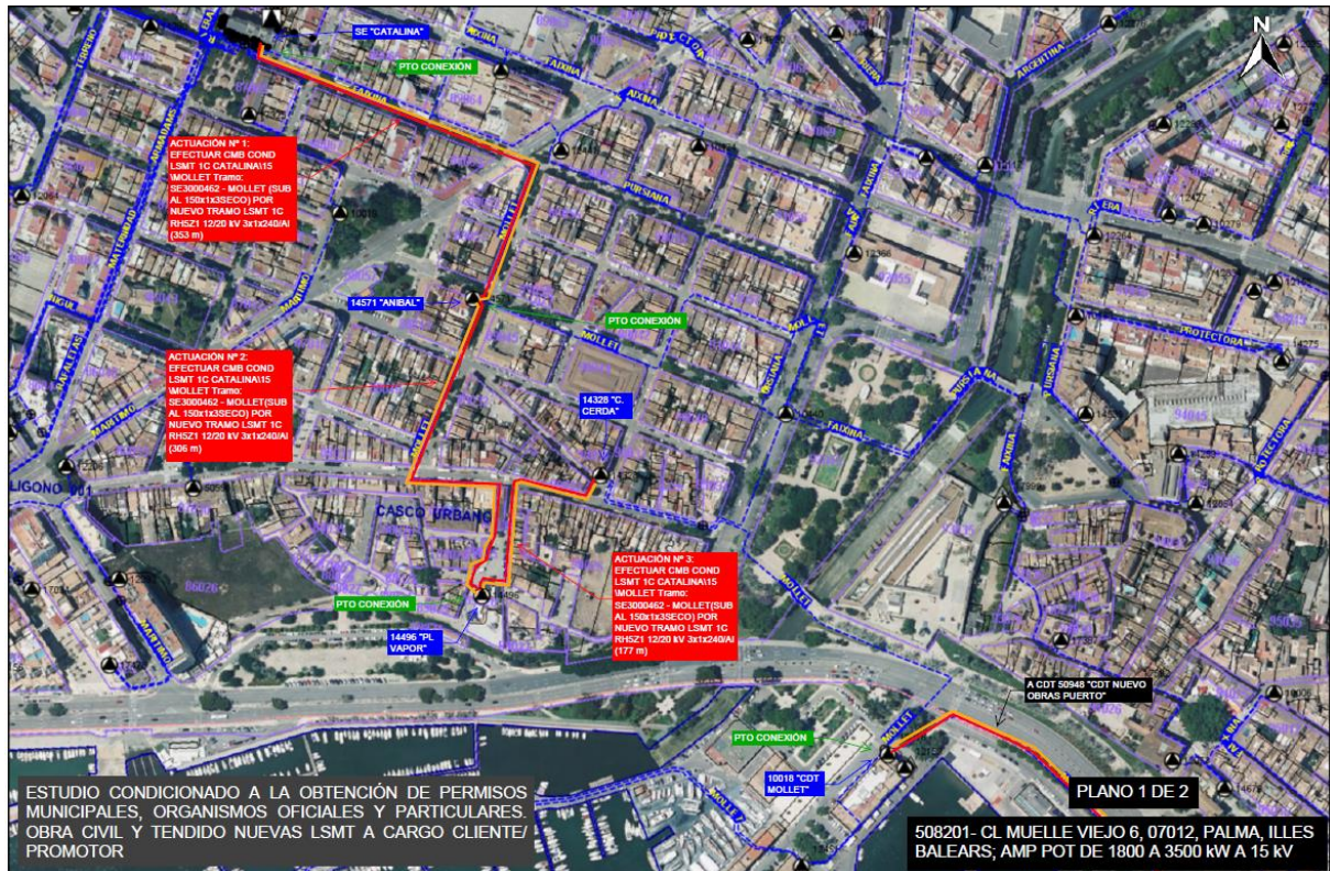
Figura 7. Actuaciones propuestas por la compañía (1 de 2) En rojo conductor existente a sustituir. En naranja nuevo conductor RH5Z1 12/20 kV 3x1x240/AI
