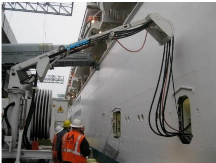
Figura 37. Reposicionar la grúa para dejar holgura en los cables de conexión
