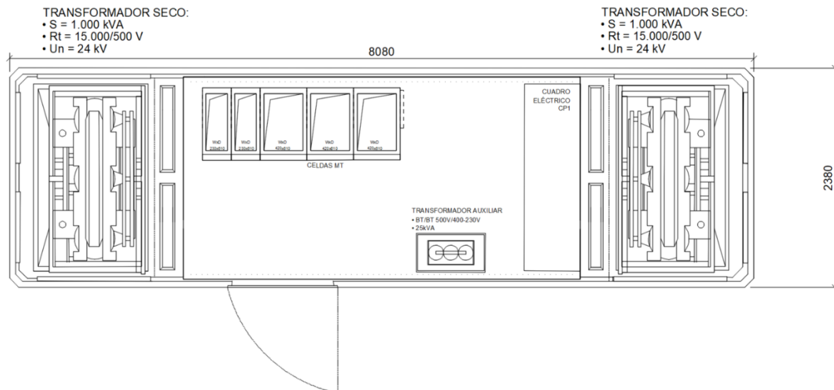
Figura 22. Planta orientativa Centro de Transformación CT-OPS
