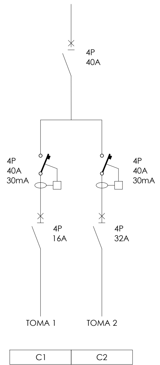
ESQUEMA ELÉCTRICO TORRETA
