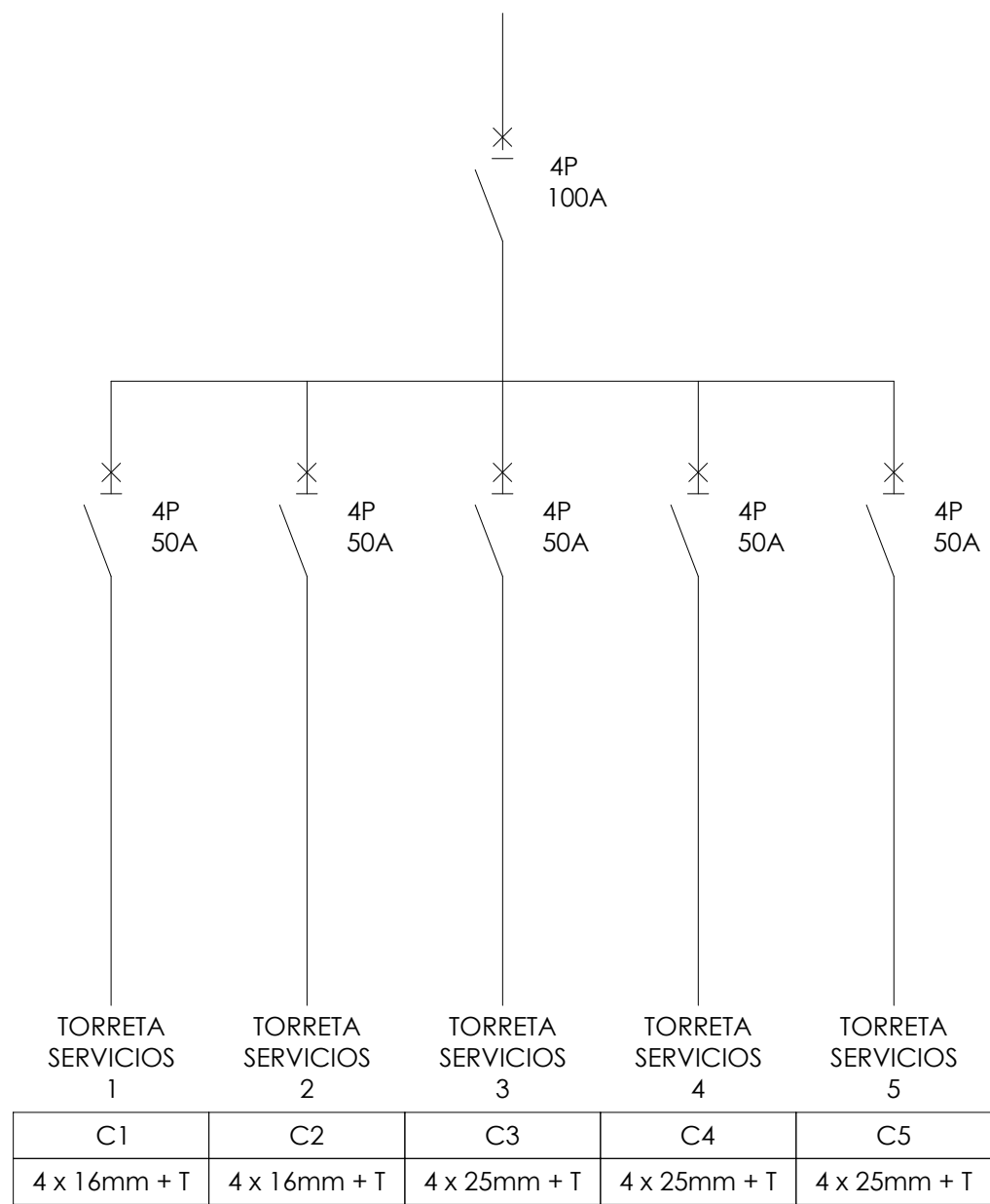
MODIFICACIÓN CUADRO ELÉCTRICO ESTACIÓN MARÍTIMA
