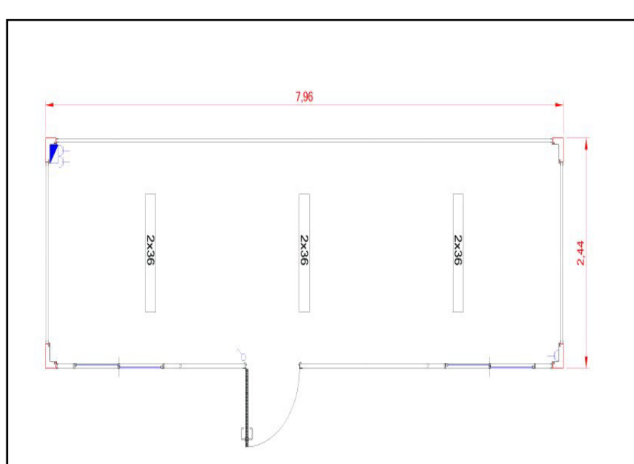
CASETA COMEDOR TIPO
