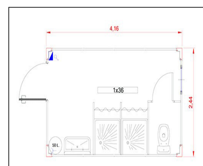
CASETA ASEO/VESTUATIO TIPO
