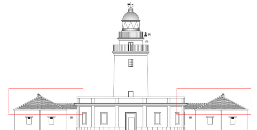
Fig. 1 Alzado del Faro
