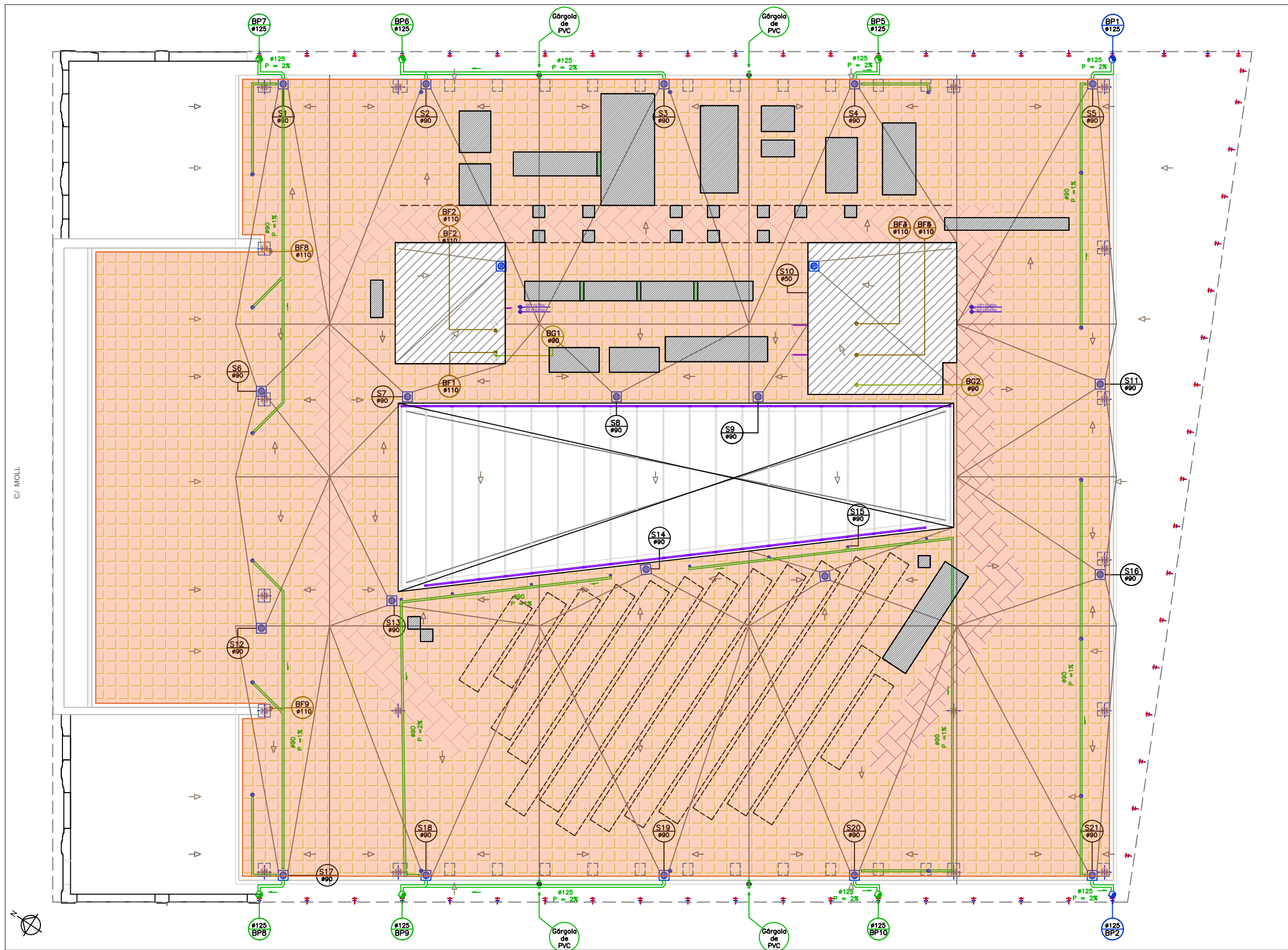
PLANTA CUBIERTA A1 1:200
