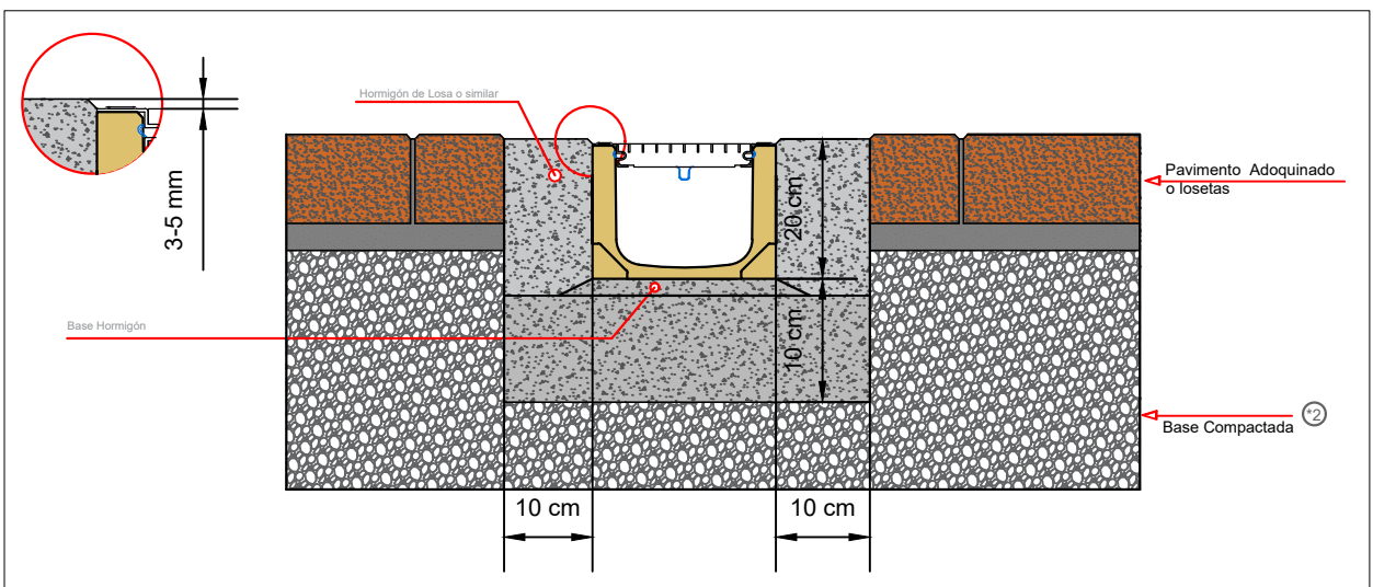
DETALLE CANALETA PREFABRICADA DE HORMIGÓN PARA DRENAJE SIN ESCALA
