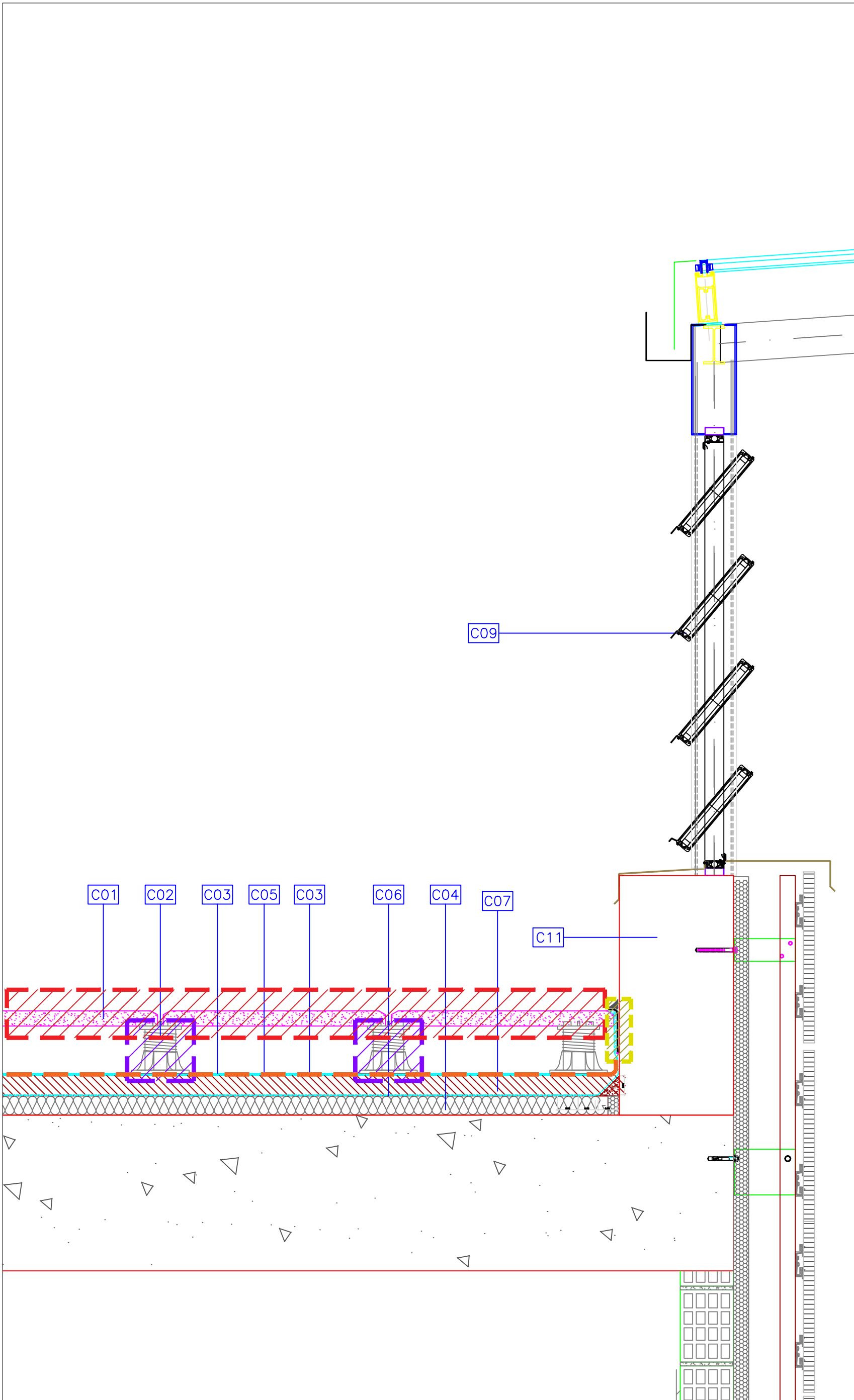
DETALLE 2 // RETIROS Y DESMONTES A1 1:10 A3 1:20
