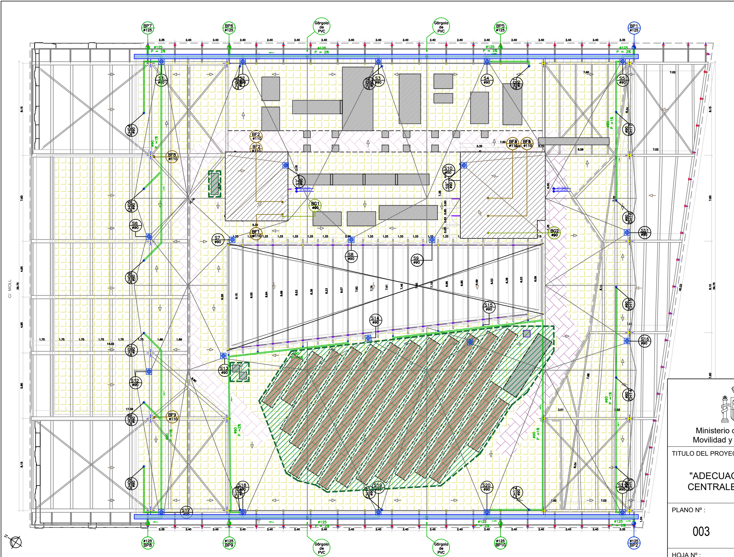
PLANTA CUBIERTA A1 1:200
