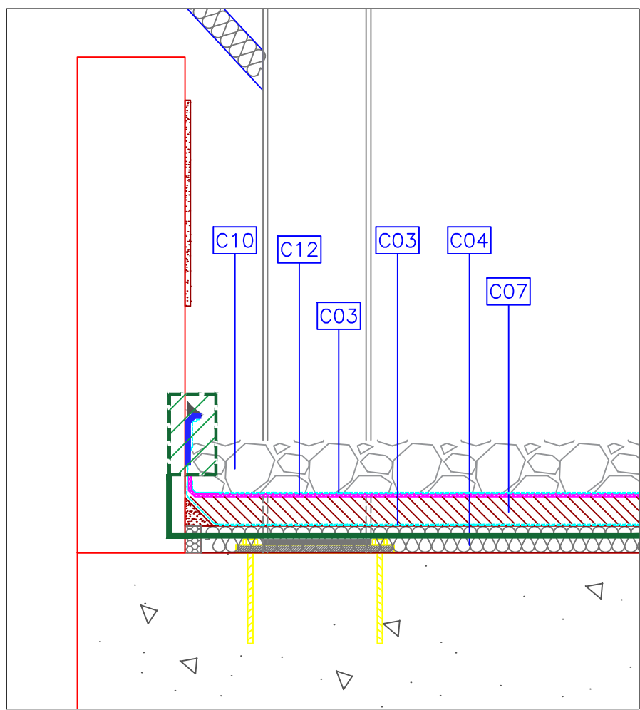
DETALLE 1 // ACTUACIÓN A1 1:10 A3 1:20
