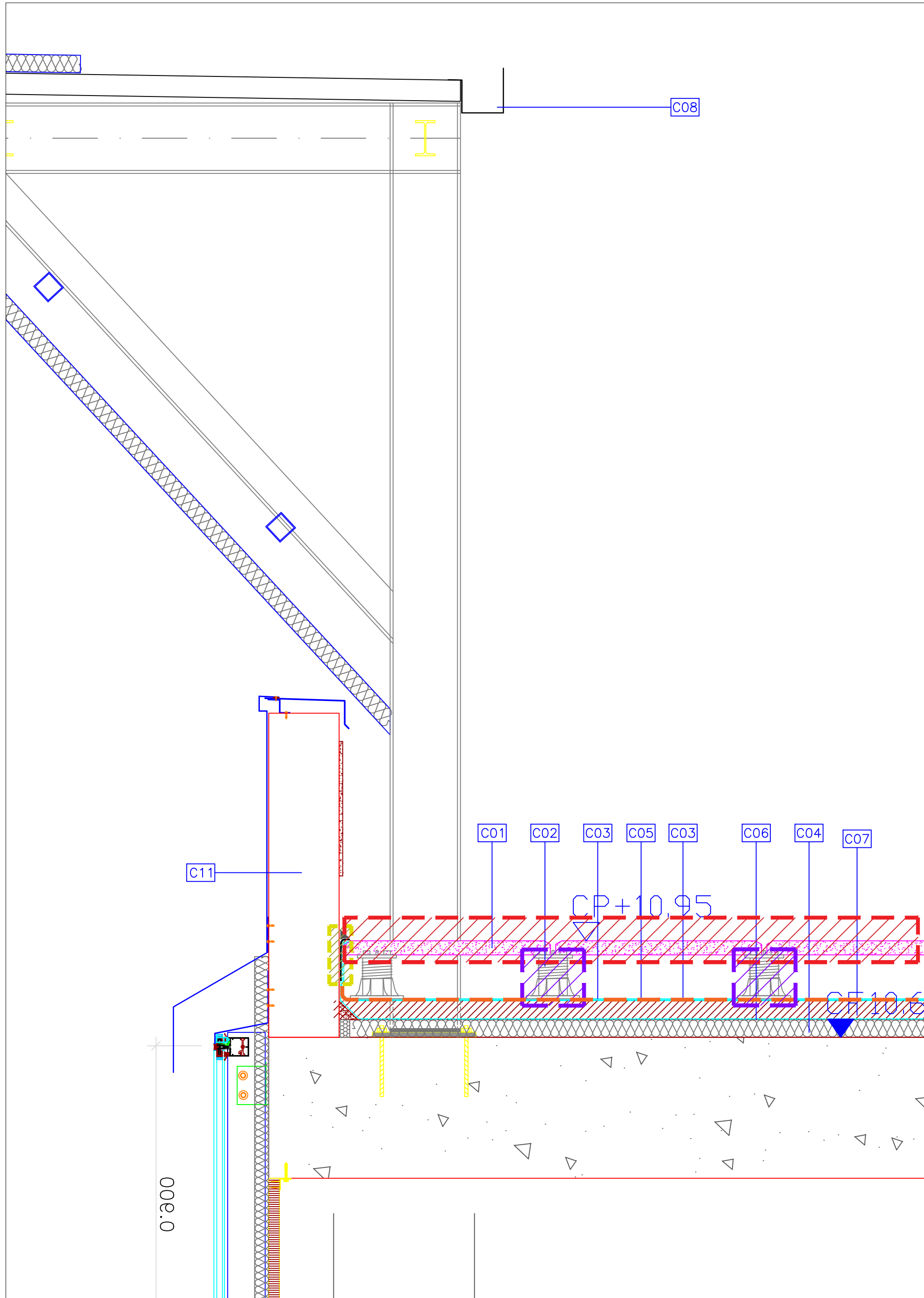
DETALLE 1 // RETIROS Y DESMONTES A1 1:10 A3 1:20
