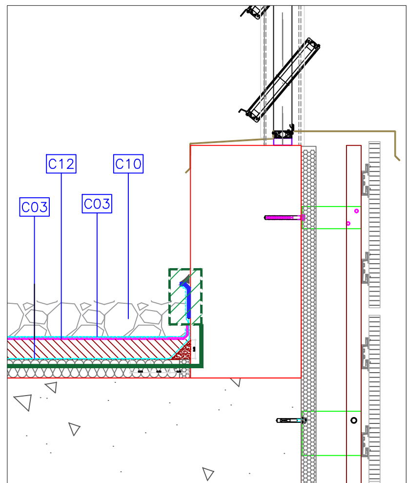
DETALLE 2 // ACTUACIÓN A1 1:10 A3 1:20
