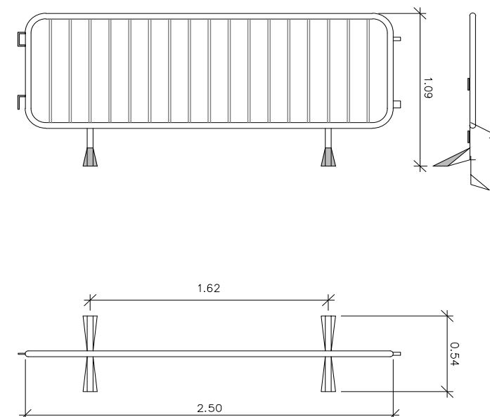
DETALLE 2. VALLA MOVIL DE PROTECCIÓN
